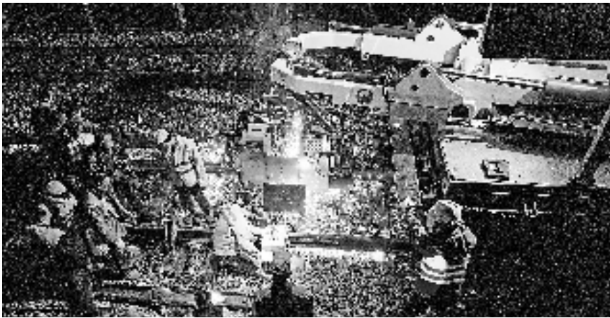
近日凌晨,工人对沪昆铁路钢轨进行换轨施工迎春运。据新华社
